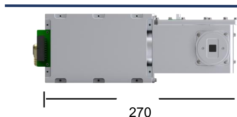
侧视图
